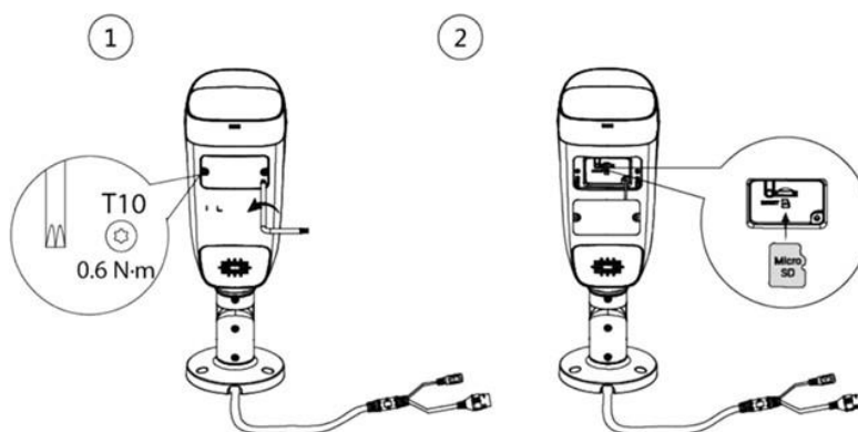
Figura 3-2 Installazione di una scheda SD (unità: mm[pollici])
