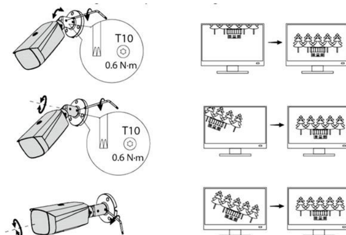
Figura 3.5 Regolazione dell'angolo dell'obiettivo
