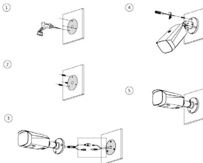
Figura 3.3 A - Passaggio del cavo attraverso la superficie di montaggio
