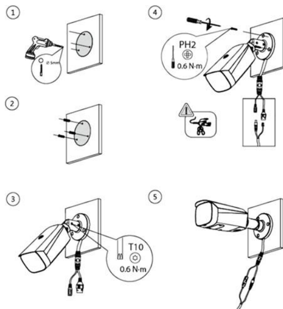
Figura 3.4 B - Passaggio del cavo attraverso la canalina laterale
