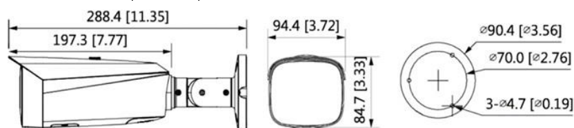
Figura 3-1 Dimensioni (unità: mm [pollici])
