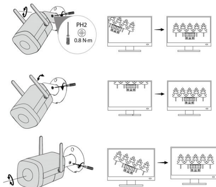
Figura 3.5 Regolazione dell'angolo dell'obiettivo
