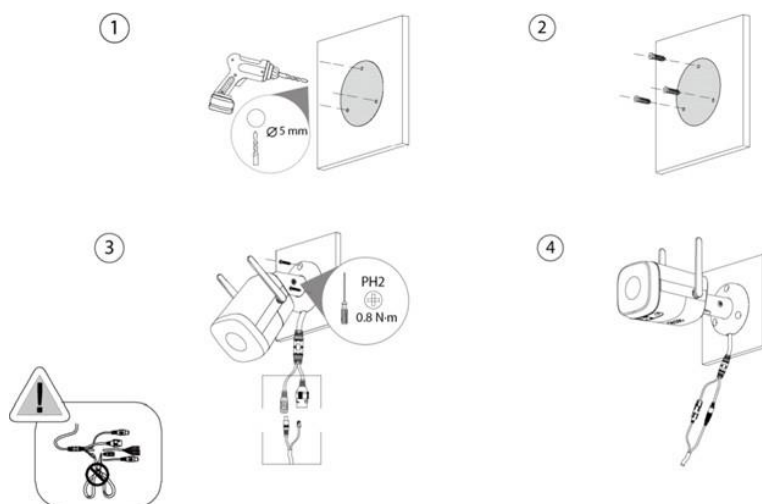
Figura 3.4 B - Passaggio del cavo attraverso la canalina laterale
