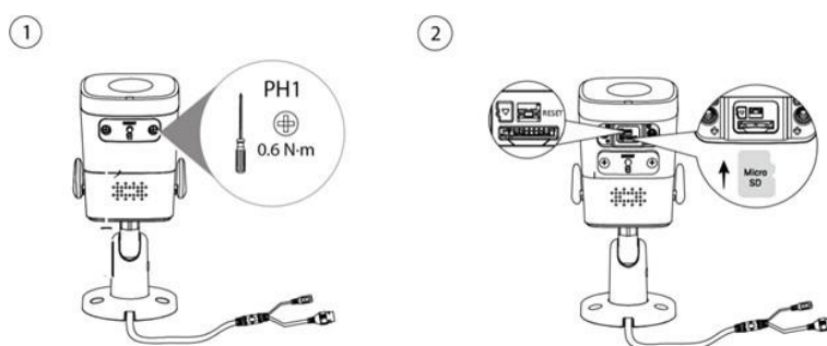
Figura 3-2 Installazione di una scheda SD (unità: mm[pollici])
