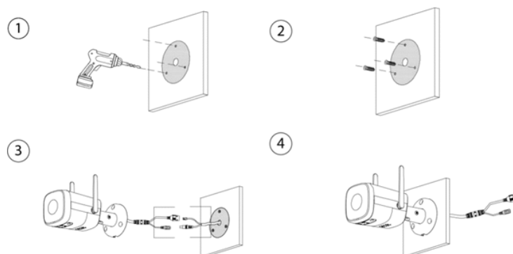
Figura 3.3 A - Passaggio del cavo attraverso la superficie di montaggio
