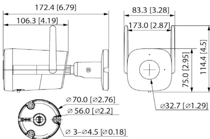
Figura 3-1 Dimensioni (unità: mm)
